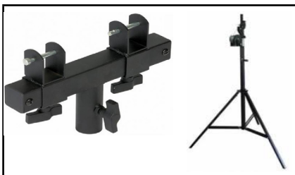
Pied à treuil MTS 410 Longueur plié: 1,74m Charge max 80kg L'unité 22,50€ H.T L'unité 27,00€ T.T.C
