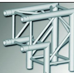
Angle 90° structure carré Diamètre du tube: 35mm L'unité 16,67€ H.T L'unité 20,00€ T.T.C
