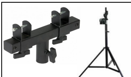
Pied à treuil MTS 270 Trépied métal hauteur max 2.7m Charge 60kg L'unité 15,00€ H.T L'unité 18,00€ T.T.C
